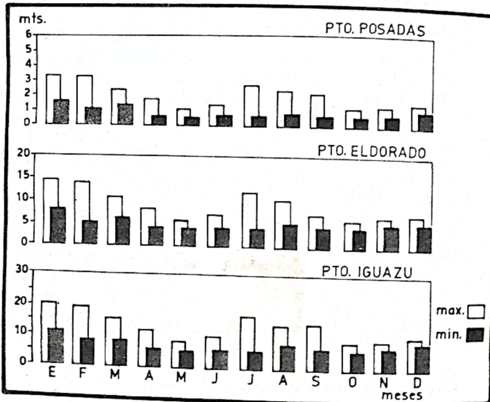
20. 2. d.- EVOLUCION DE LAS ALTURAS MAXIMA Y MINIMA DE LOS RIOS PARANA E IGUAZU, REGISTRADAS MENSUALMENTE EN LOS PUERTOS DE POSADAS, ELDORADO E IGUAZU - AÑO 1978
