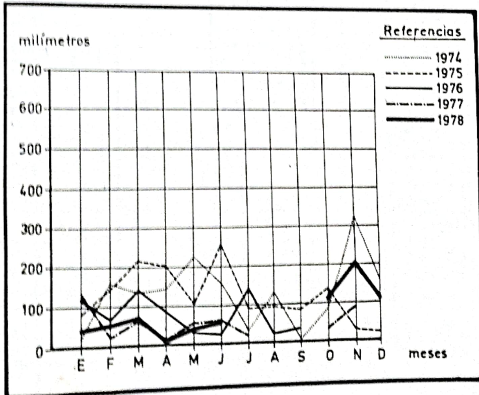
20. 1. f.- EVOLUCION DE LAS PRECIPITACIONES REGISTRADAS EN LA LOCALIDAD DE CAMPO VIERA, POR MES 1974 - 1978 ( en mm.)
