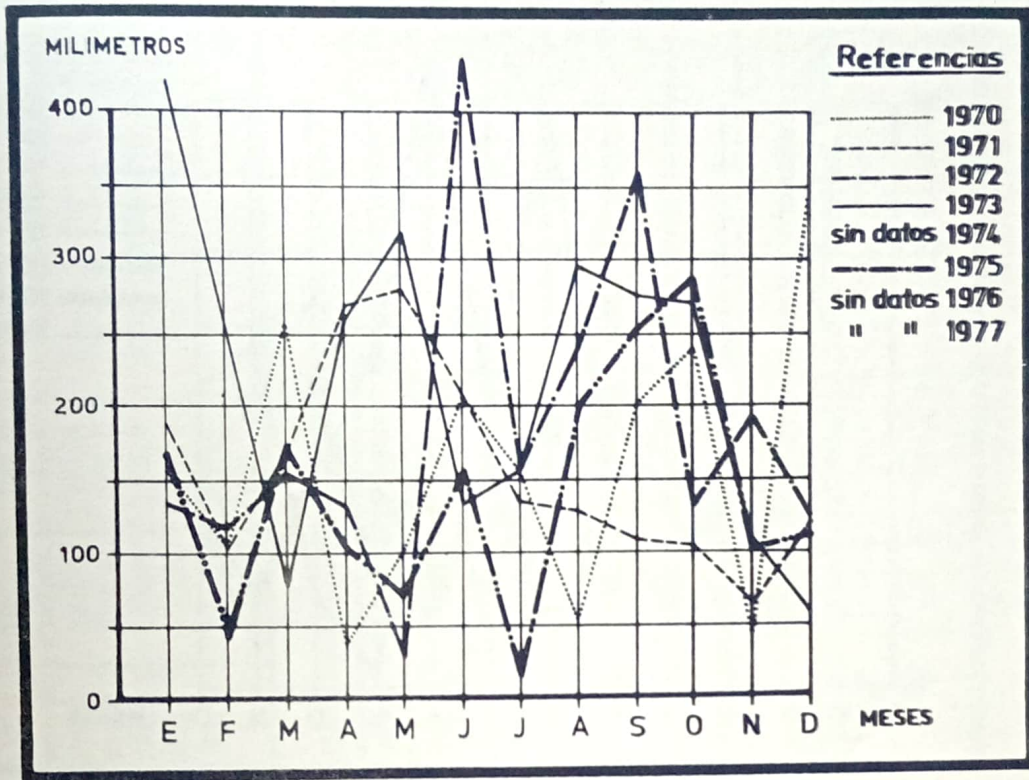
20.1.1. - EVOLUCION DE LAS PRECIPITACIONES REGISTRADAS EN LA LOCALIDAD DE SAN ANTONIO, POR MES. - 1970 - 1977 (en mm.)
