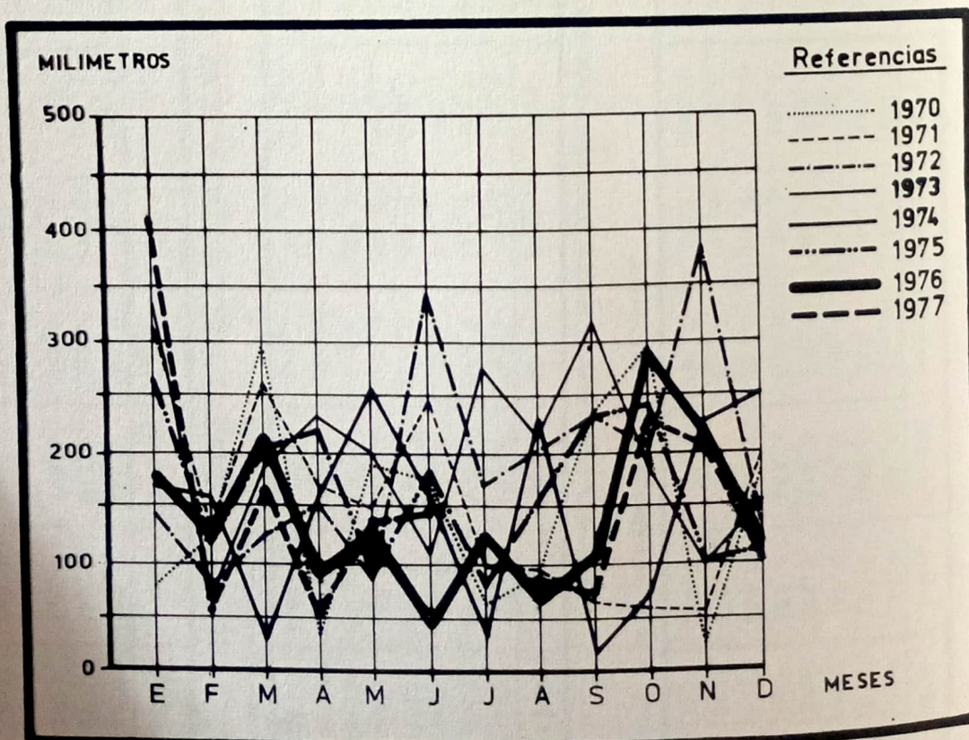
20.1.b. - PRECIPITACIONES REGISTRADAS EN LA LOCALIDAD DE SANTO PIPO POR MES. - 1970 - 1977 (en mm.)
