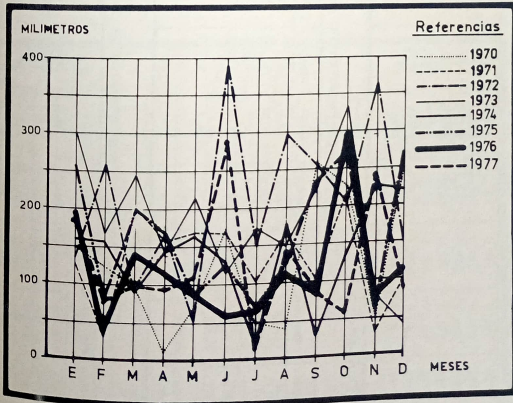
20.1.f. - EVOLUCION DE LAS PRECIPITACIONES REGISTRADAS EN LA LOCALIDAD DE ELDORADO, POR MES. - 1970 - 1977 (en mm.)
