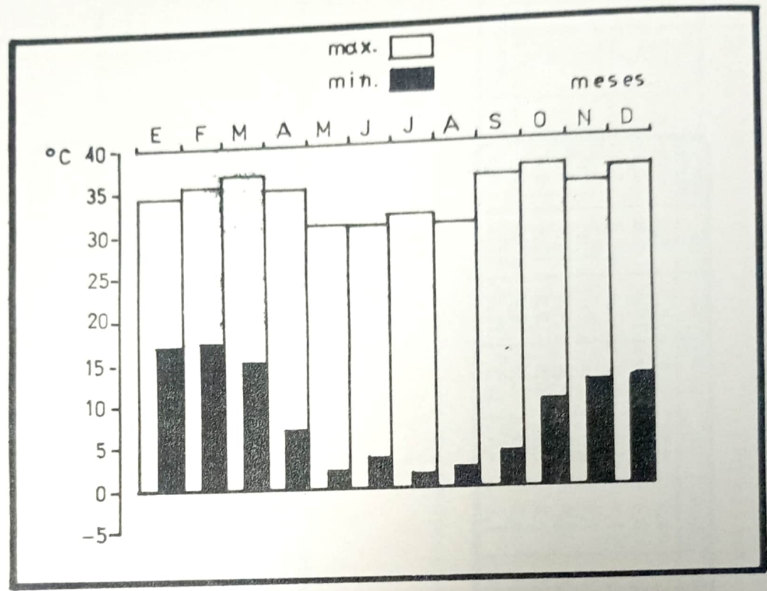
20.1.p. - TEMPERATURAS MINIMA Y MAXIMA ABSOLUTAS, REGISTRADAS EN POSADAS POR MES 1977 (EN Cº)
