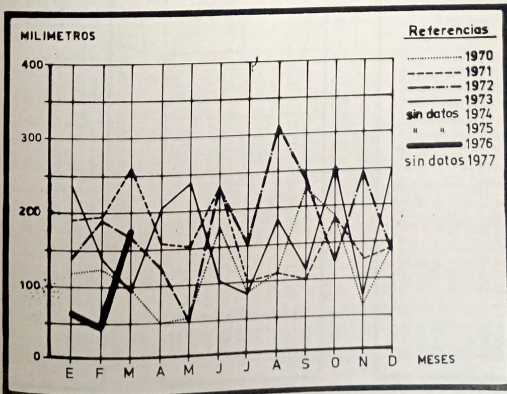
20.1.h. - EVOLUCION DE LAS PRECIPITACIONES REGISTRADAS EN LA LOCALIDAD DE IGUAZU, POR MES. - 1970 - 1977 (en mm.)
