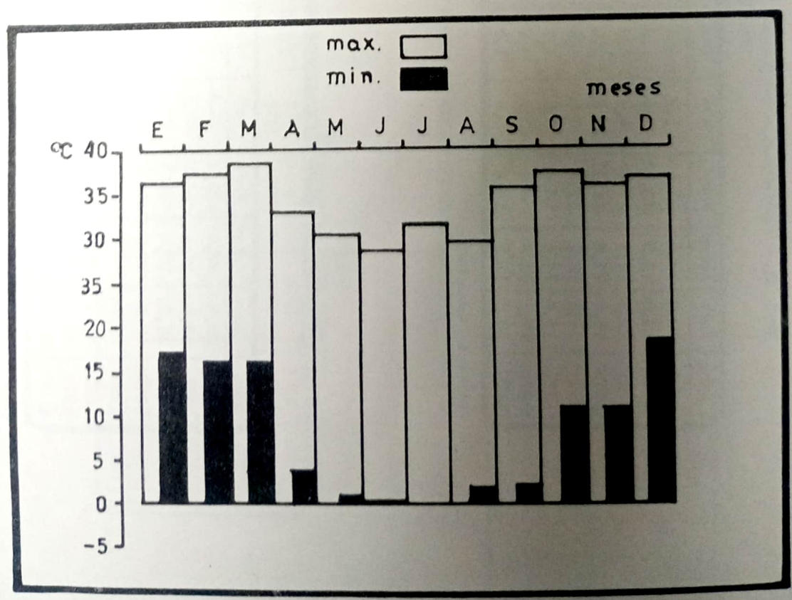
20.1.q. - TEMPERATURAS MINIMA Y MAXIMA ABSOLUTAS, REGISTRADAS EN MONTECARLO POR MES. - 1977 (Co)
