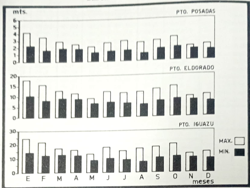
20.2.a. - EVOLUCION DE LAS ALTURAS MAXIMA Y MINIMA DE LOS RIOS PARANA E IGUAZU, REGISTRADAS MENSUALMENTE EN LOS PUERTOS DE POSADAS, ELDORADO E IGUAZU - AÑO 1973
