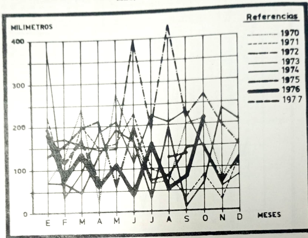
20.1.k. - PRECIPITACIONES REGISTRADAS EN LA LOCALIDAD DE CAMPO GRANDE POR MES, - 1970 - 1977 (en mm.)
