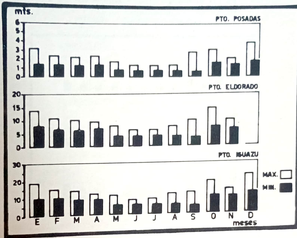
20.2.c. - EVOLUCION DE LAS ALTURAS MAXIMA Y MINIMA DE LOS RIOS PARANA E IGUAZU, REGISTRADAS MENSUALMENTE EN LOS PUERTOS DE POSADAS, ELDORADO E IGUAZU - AÑO 1975
