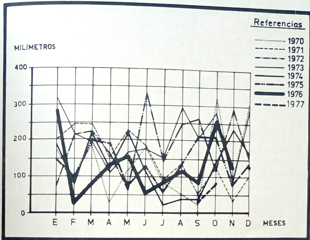
20.1.e. - EVOLUCION DE LAS PRECIPITACIONES REGISTRADAS EN LA LOCALIDAD DE PIRAY, POR MES. - 1970 - 1977 (en mm.)
