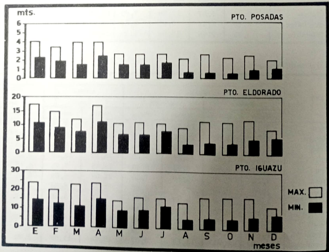
20.2.b. - EVOLUCION DE LAS ALTURAS MAXIMA Y MINIMA DE LOS RIOS PARANA E IGUAZU, REGISTRADAS MENSUALMENTE EN LOS PUERTOS DE POSADAS, ELDORADO E IGUAZU - AÑO 1974
