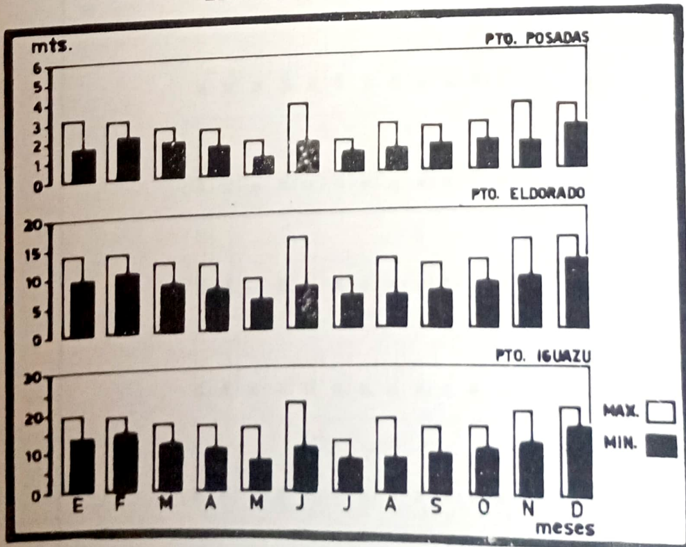
20.2.d. - EVOLUCION DE LAS ALTURAS MAXIMA Y MINIMA DE LOS RIOS PARANA E IGUAZU, REGISTRADAS MENSUALMENTE EN LOS PUERTOS DE POSADAS, ELDORADO E IGUAZU - AÑO 1976
