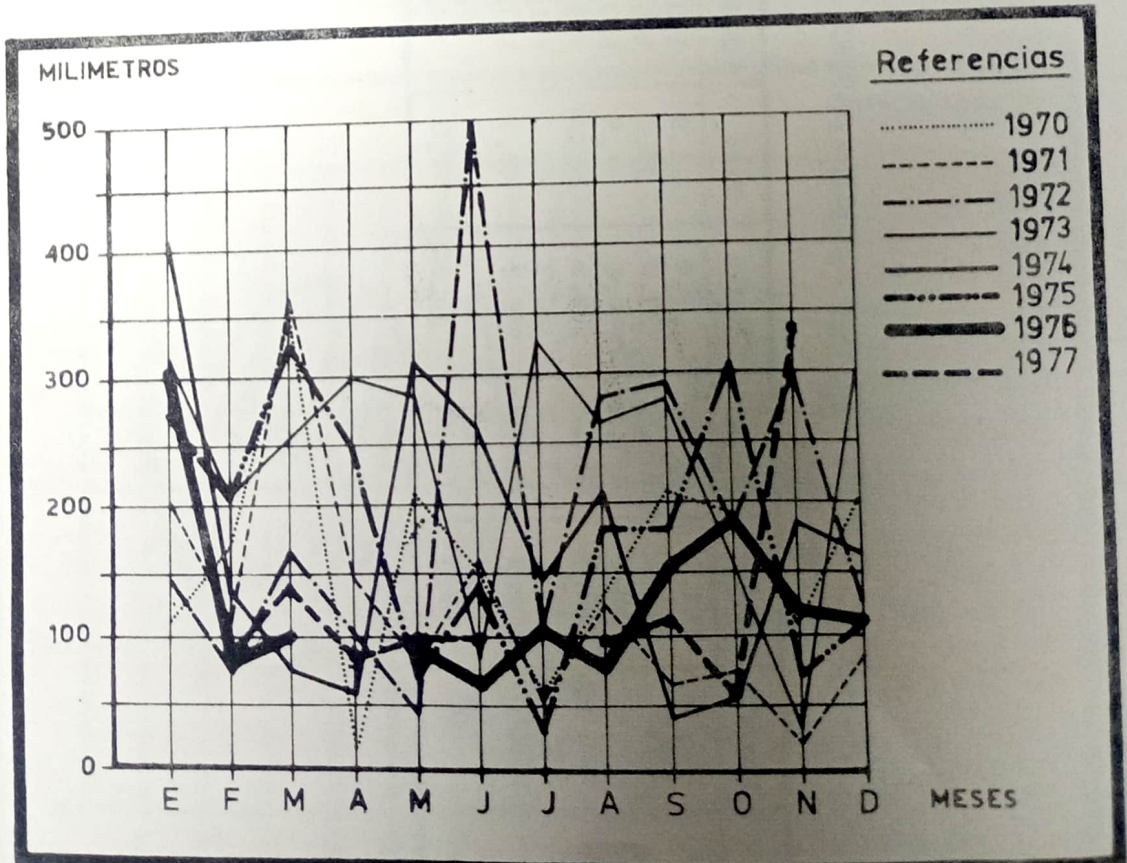
20.1.o. - EVOLUCION DE LAS PRECIPITACIONES REGISTRADAS EN LA LOCALIDAD DE APOSTOLES, POR MES. - 1970 - 1977 (en mm.)
