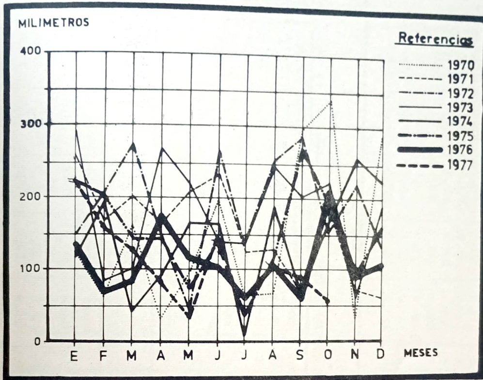
20.1.g. - EVOLUCION DE LAS PRECIPITACIONES REGISTRADAS EN LA LOCALIDAD DE ESPERANZA, POR MES. - 1970 - 1977-
