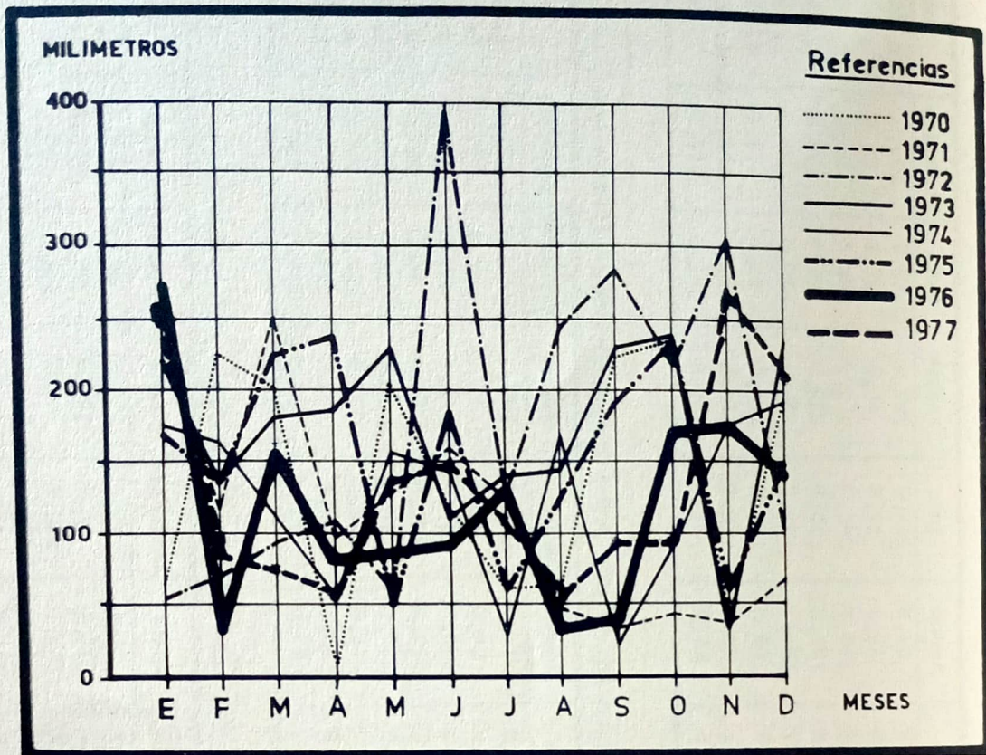
20.1.a. - EVOLUCION DE LAS PRECIPITACIONES REGISTRADAS EN LA LOCALIDAD DE POSADAS, POR MES. - 1970 - 1977 (en mm.)
