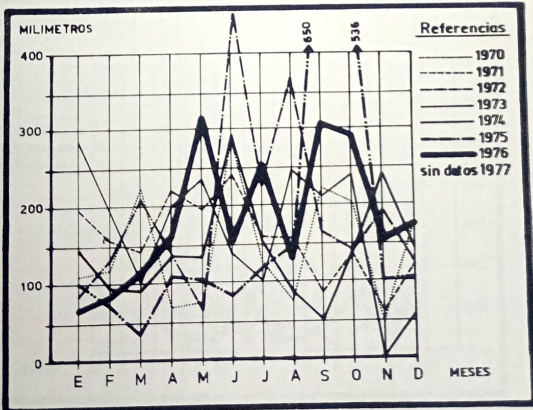
20.1.j. - EVOLUCION DE LAS PRECIPITACIONES REGISTRADAS EN LA LOCALIDAD DE BERNARDO DE IRIGOYEN, POR MES. - 1970 - 1977 (en mm.)
