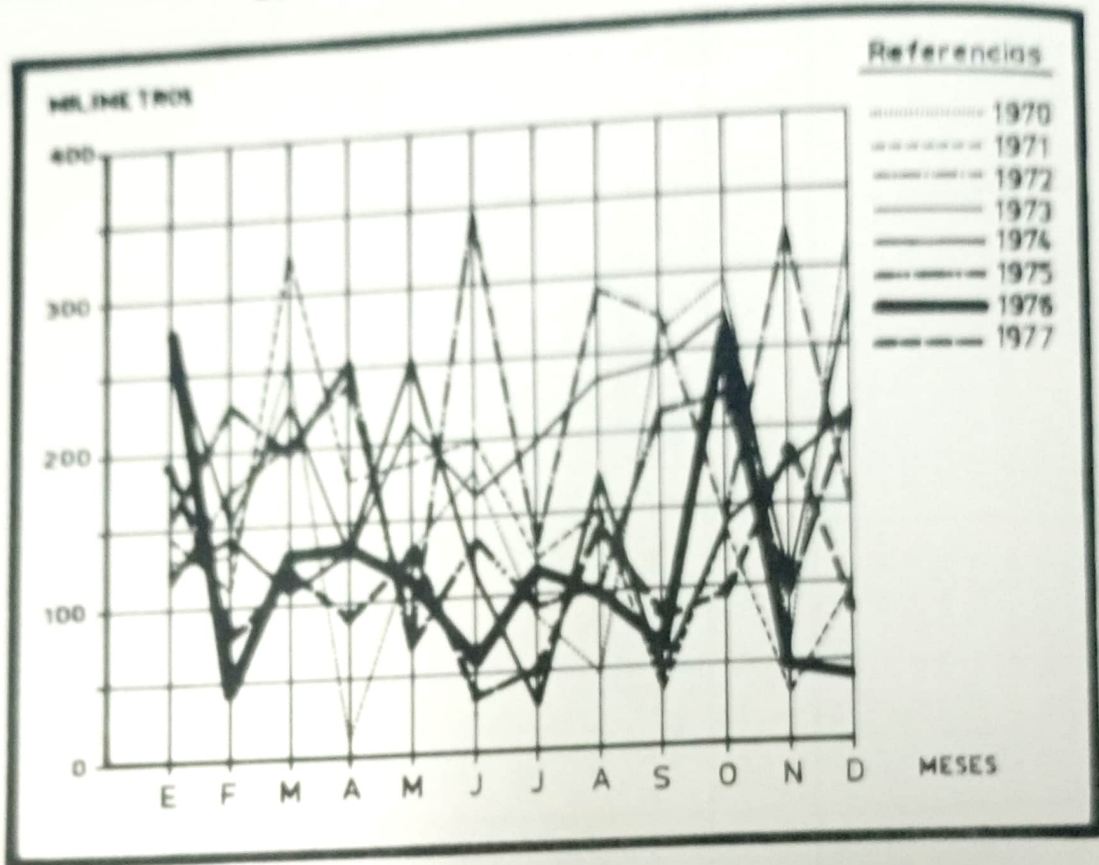
20.1.c. - EVOLUCION DE LAS PRECIPITACIONES REGISTRADAS EN LA LOCALIDAD DE MONTECARLO POR MES. - 1970 - 1977 (en mm.)
