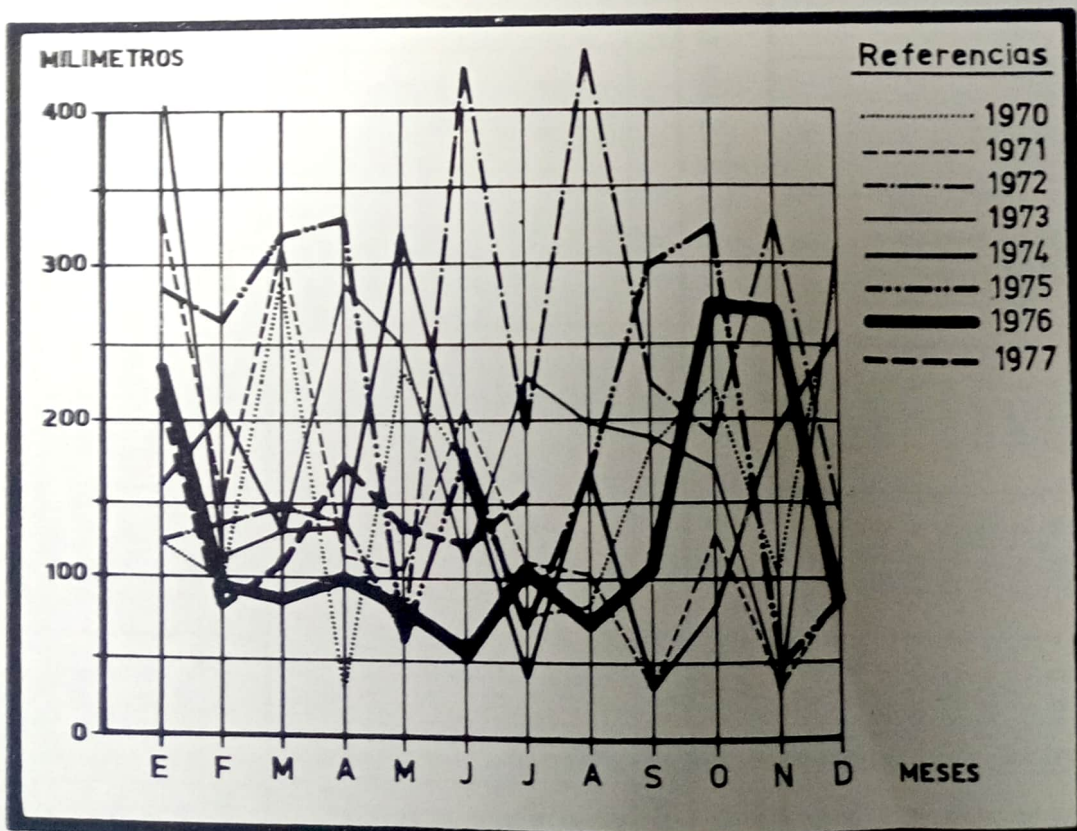
20.1.n. - EVOLUCION DE LAS PRECIPITACIONES REGISTRADAS EN LA LOCALIDAD DE CERRO AZUL POR MES. - 1970 - 1977 (en mm.)
