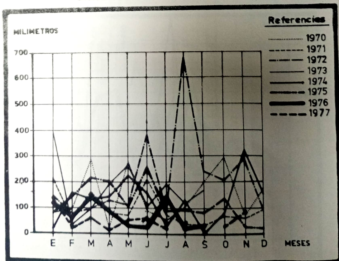
20.1.l - EVOLUCION DE LAS PRECIPITACIONES REGISTRADAS EN LA LOCALIDAD DE CAMPO VIERA POR MES, - 1970 - 1977 (en mm.)
