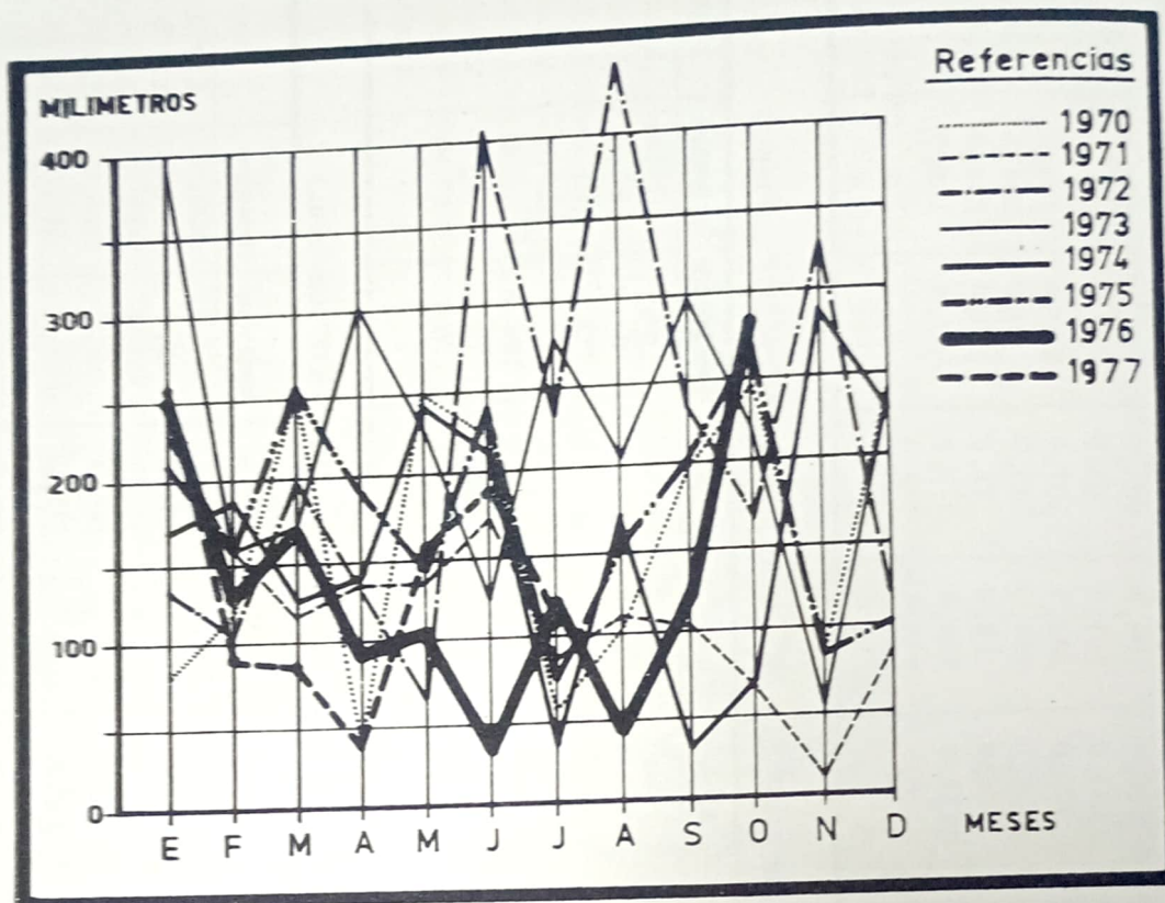
20.1.m. - EVOLUCION DE LAS PRECIPITACIONES REGISTRADAS EN LA LOCALIDAD DE OBERA, POR MES. - 1970 - 1977 (en mm.)
