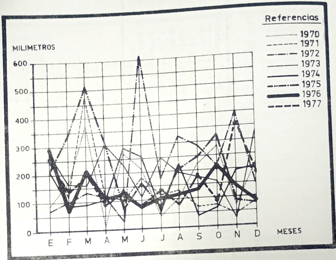
20.1.a. - EVOLUCION DE LAS PRECIPITACIONES REGISTRADAS EN LA LOCALIDAD DE SAN JOSE, POR MES. - 1970 - 1977 (en mm.)
