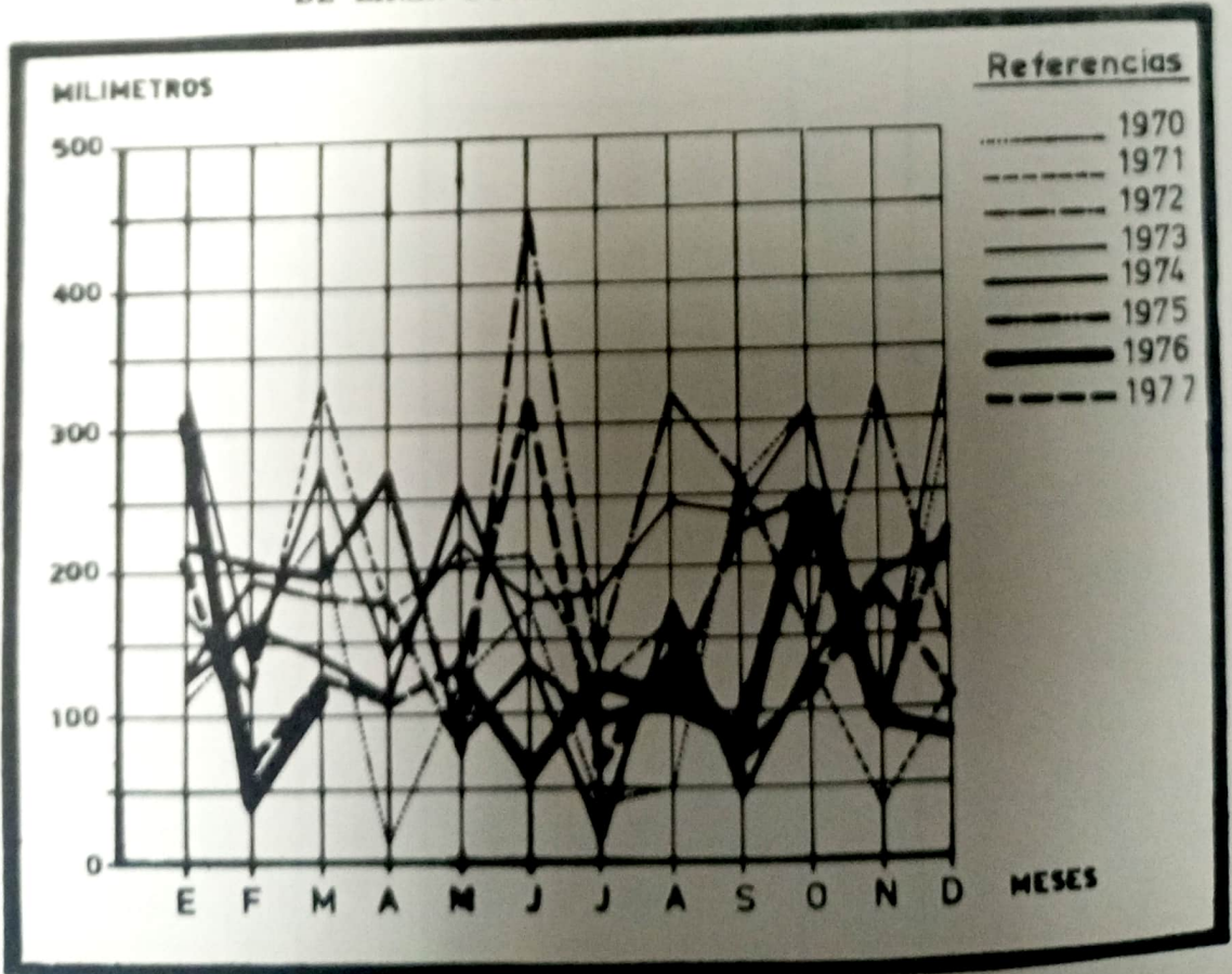
20.1.d. - EVOLUCION DE LAS PRECIPITACIONES REGISTRADAS EN LA LOCALIDAD DE LINEA BONITA POR MES. - 1970 - 1977 (en mm.)
