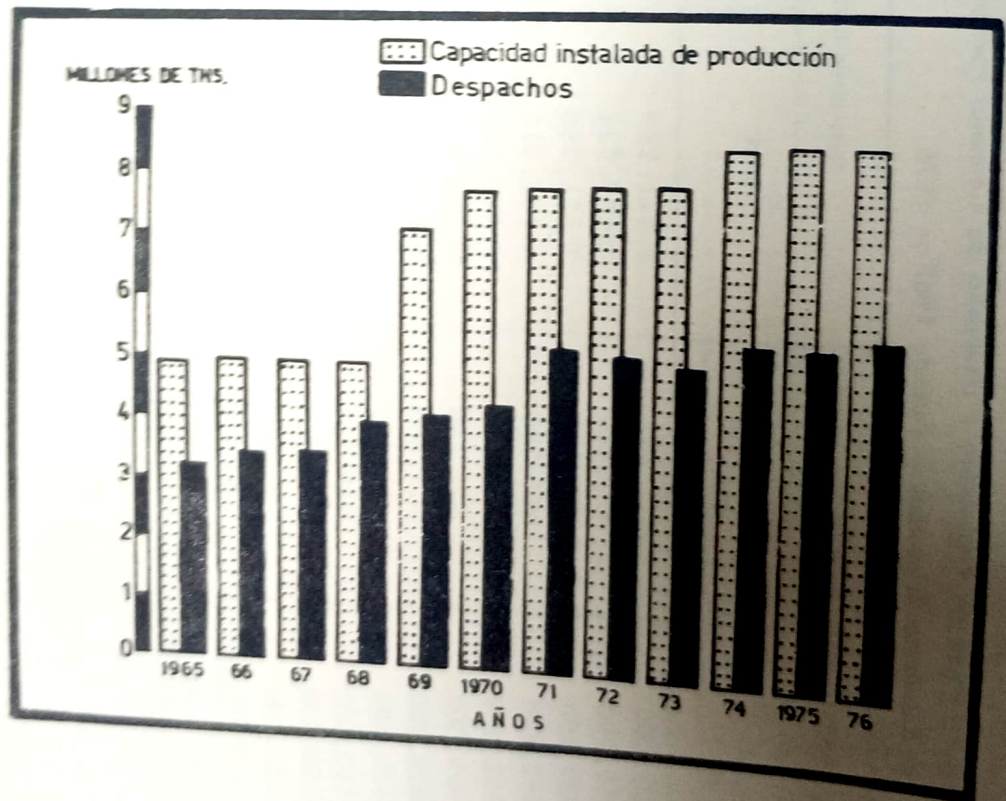
12 a. - Evolución de la Capacidad Instalada de Producción y Despachos de Cemento Portland en la República Argentina - Período 1965 - 1976
