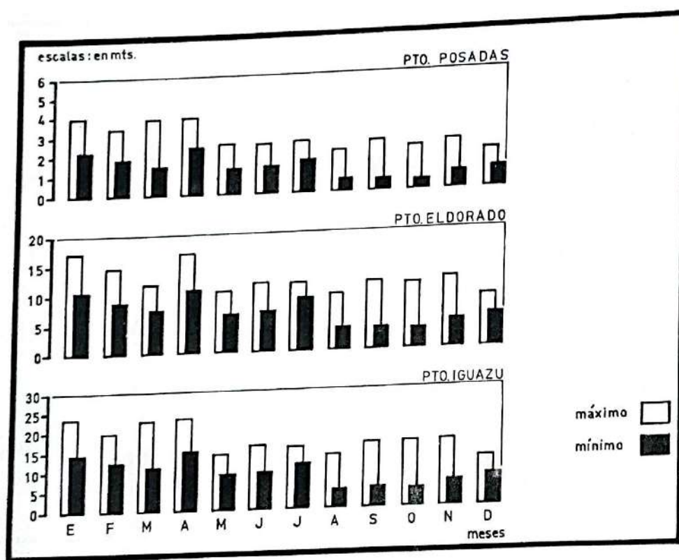
20.2.b. - EVOLUCION DE LAS ALTURAS MAXIMAS Y MINIMA DEL RIO PARANA, REGISTRADAS MENSUALMENTE EN LOS PUERTOS DE POSADAS, EL - DORADO E IGUAZU -AÑO 1974.-
