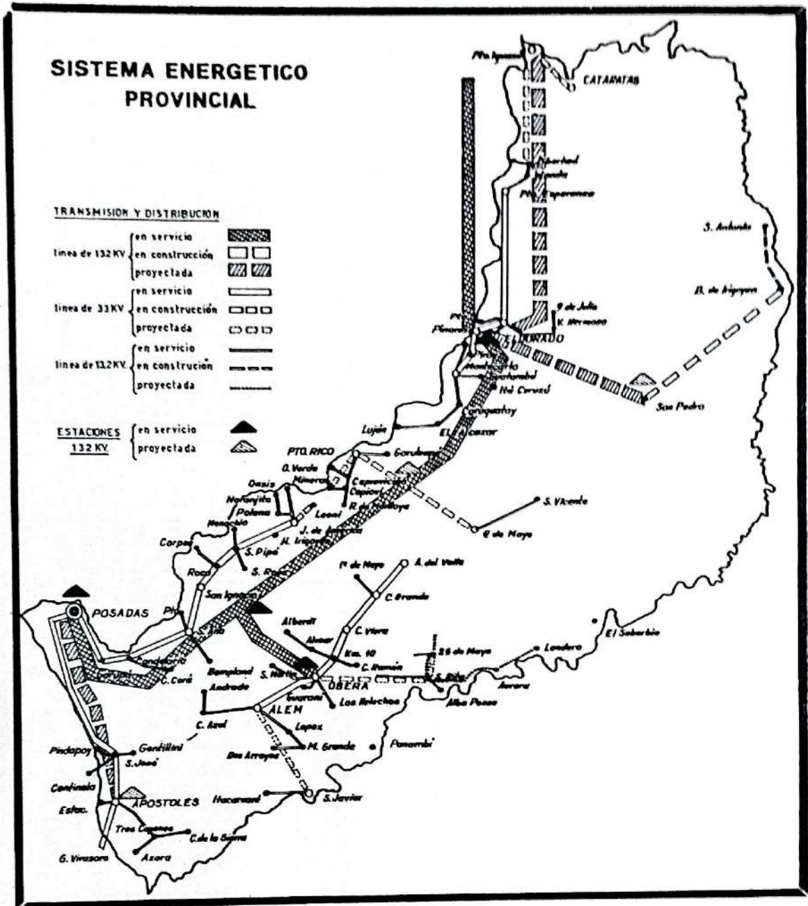
14. a. - SISTEMA ENERGETICO DE LA PROVINCIA DE MISIONES, 1974 . -
