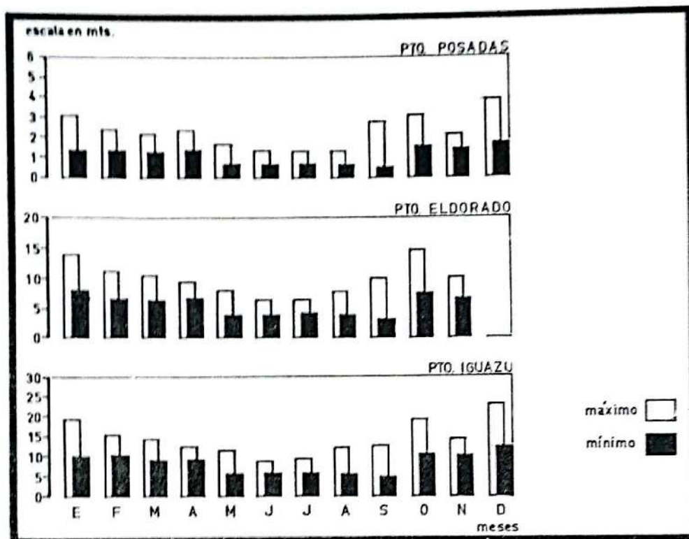
20.2.c.- EVOLUCION DE LAS ALTURAS MAXIMA Y MINIMA DEL RIO PARANA, REGISTRADAS MENSUALMENTE EN LOS PUERTOS DE POSADAS, EL DORADO E IGUAZU - AÑO 1975.-
