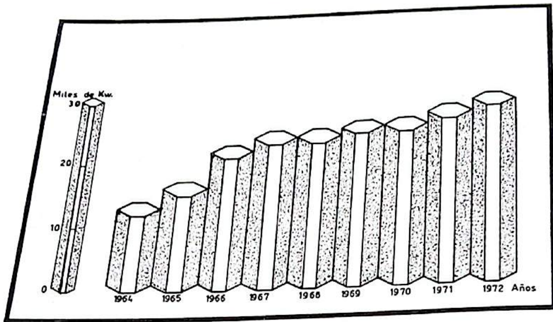
14.a- Evolución de la potencia instalada en la Provincia de Misiones Período 1964-1972
