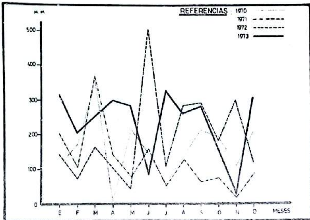
20.o.- EVOLUCION DE LAS PRECIPITACIONES REGISTRADAS EN LA LOCALIDAD DE APOSTOLES, POR MES - 1970-1973 -EN M M
