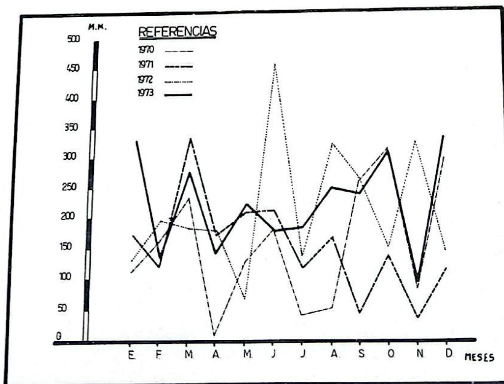
20.d.- EVOLUCION DE LAS PRECIPITACIONES REGISTRADAS EN LA LOCALIDAD DE LINEA BONITA, POR MES - 1970-1973 EN M M
