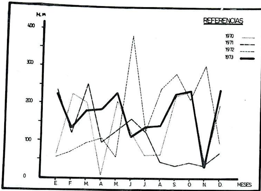
20.a.- EVOLUCION DE LAS PRECIPITACIONES REGISTRADAS EN LA LOCALIDAD DE POSADAS, POR MES - 1970-1973 - EN M M
