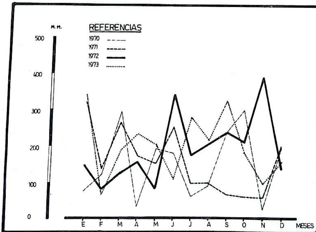
20.b.- EVOLUCION DE LAS PRECIPITACIONES REGISTRADAS EN LA LOCALIDAD DE SANTO PIPO, POR MES - 1970-1973 - EN M M
