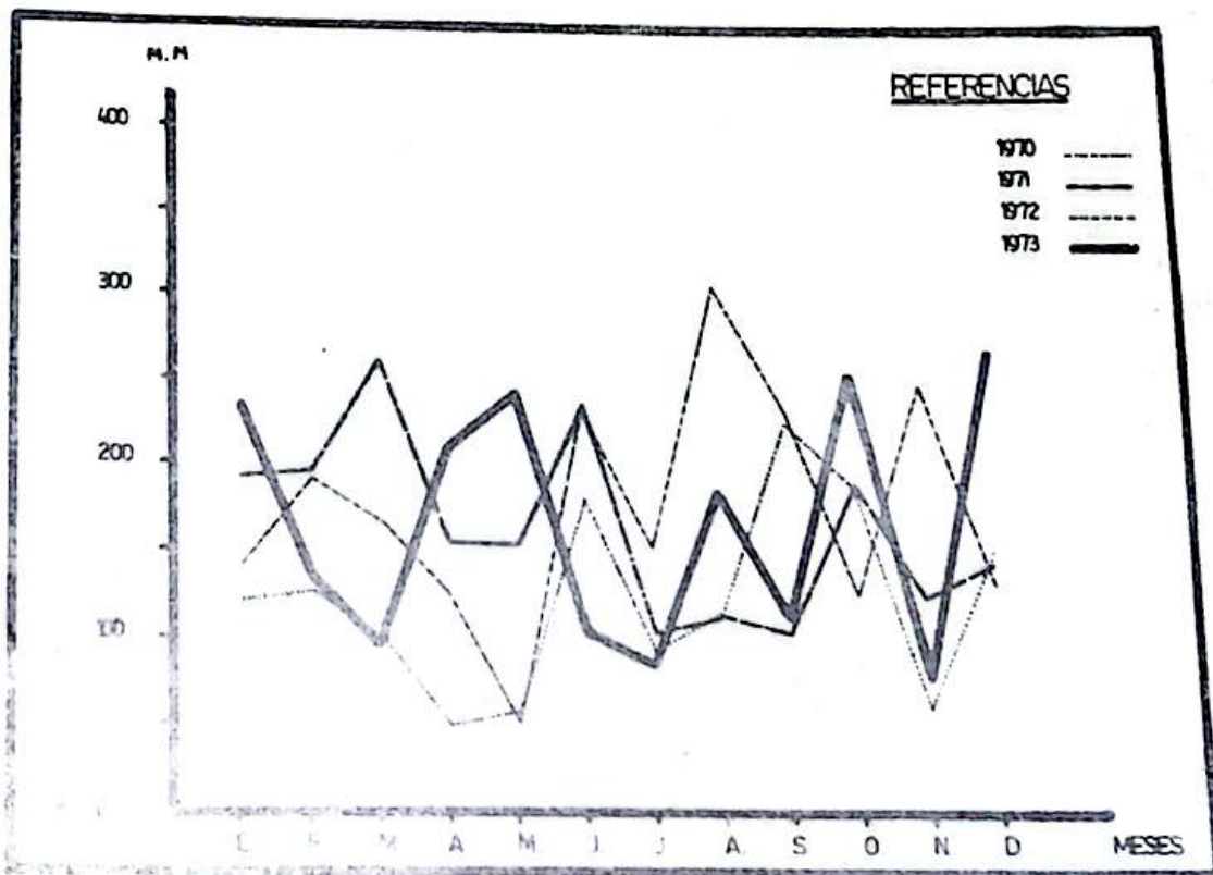
20.h.- EVOLUCION DE LAS PRECIPITACIONES REGISTRADAS EN LA LOCALIDAD DE IGUAZU, POR MES - 1970-1973 - EN M M
