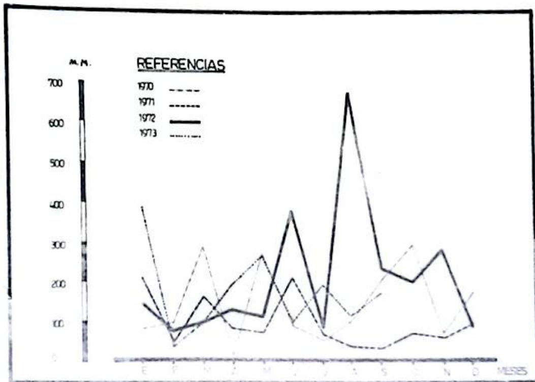
20.L- EVOLUCION DE LAS PRECIPITACIONES REGISTRADAS EN LA LOCALIDAD DE CAMPO VIERA, POR MES - 1970-1973 -EN M M
