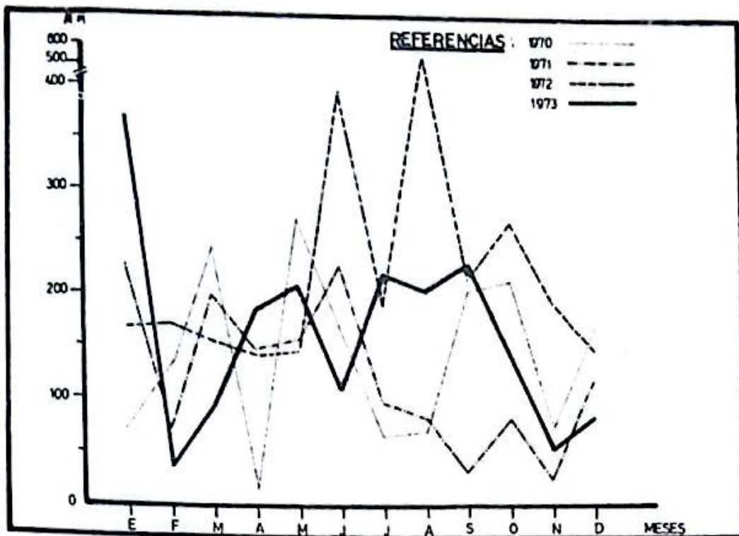
20.L- EVOLUCION DE LAS PRECIPITACIONES REGISTRADAS EN LA LOCALIDAD DE CAMPO VIERA, POR MES - 1970-1973 -EN M M
