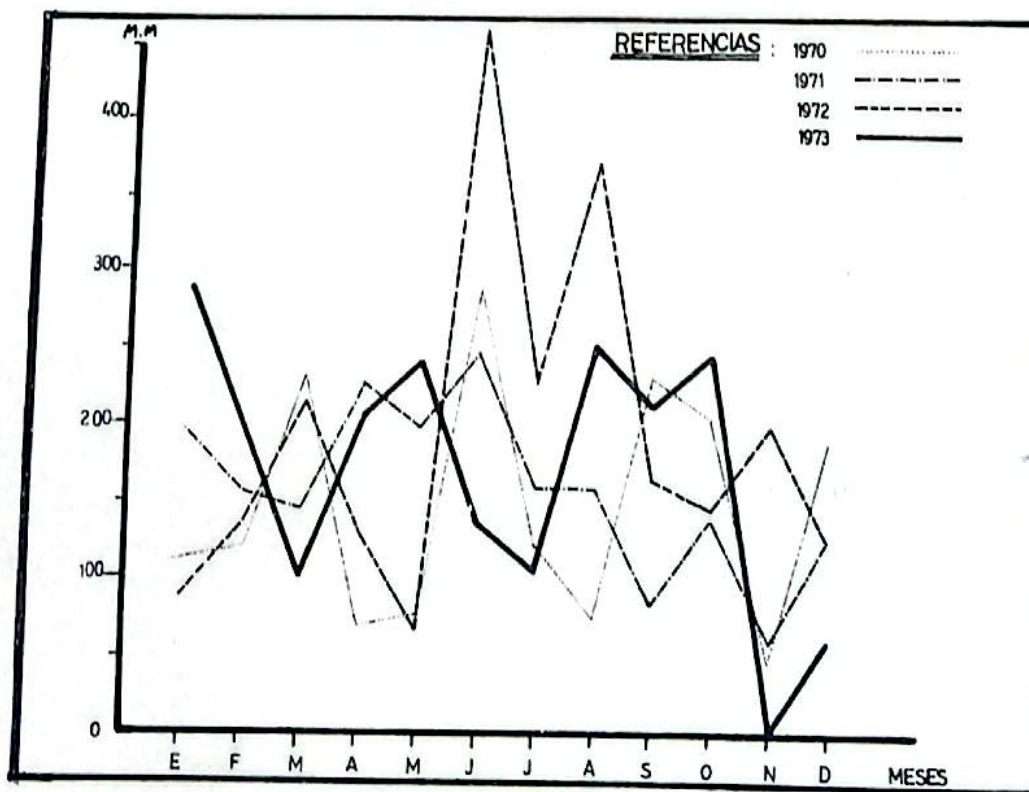
20.J.- EVOLUCION DE LAS PRECIPITACIONES REGISTRADAS EN LA LOCALIDAD DE BERNARDO DE IRIGOYEN, POR MES - 1970-1973- EN M M
