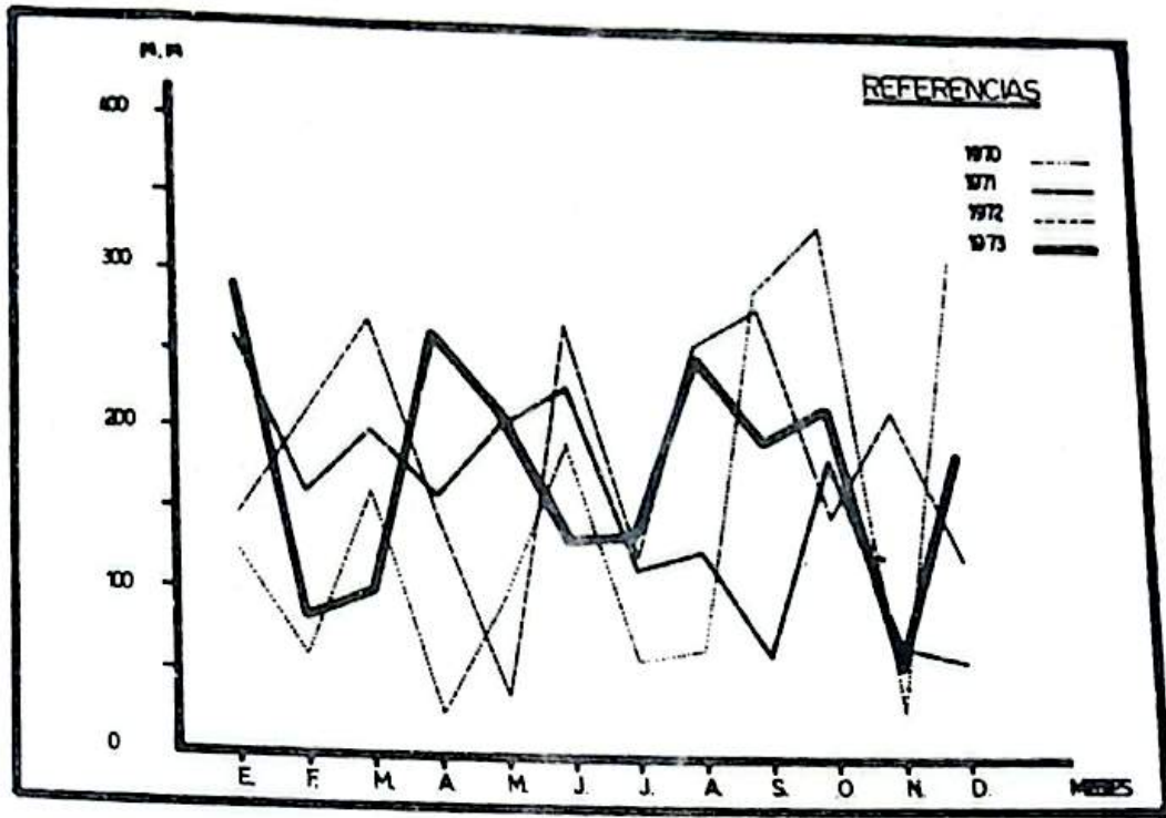
20.g.- EVOLUCION DE LAS PRECIPITACIONES REGISTRADAS EN LA LOCALIDAD DE ESPERANZA, POR MES - 1970-1973 - EN M M
