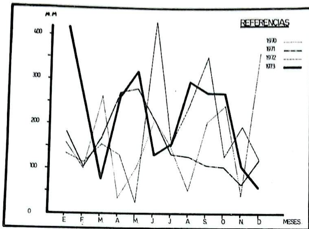
20.J.- EVOLUCION DE LAS PRECIPITACIONES REGISTRADAS EN LA LOCALIDAD DE BERNARDO DE IRIGOYEN, POR MES - 1970-1973- EN M M
