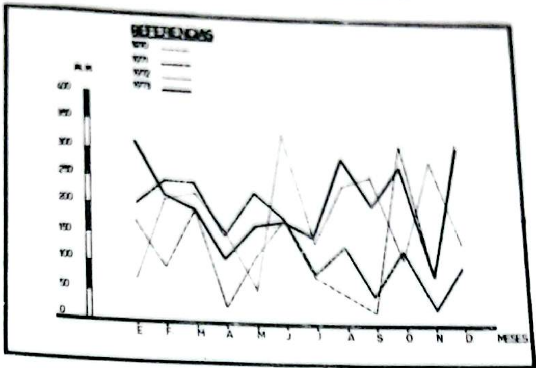
20.A.- EVOLUCION DE LAS PRECIPITACIONES REGISTRADAS EN LA LOCALIDAD DE ENRAY, POR MES - 1970-1973 - EN M M
