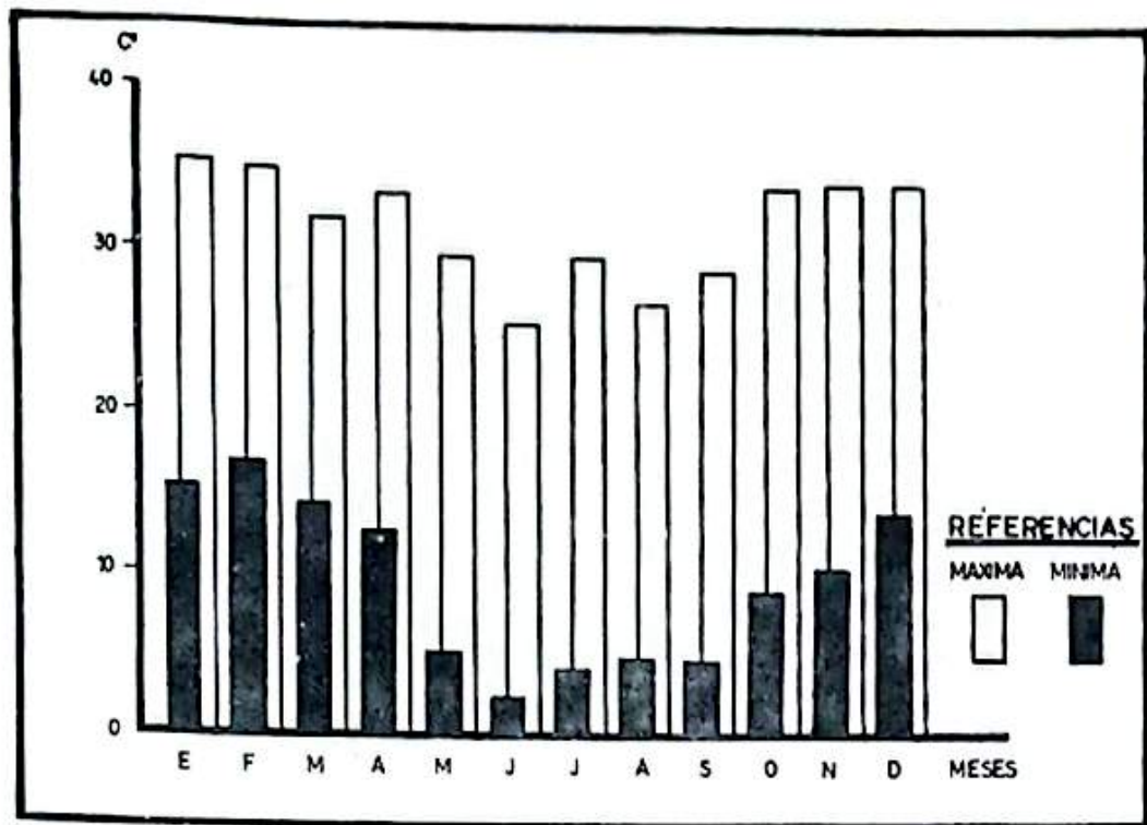
20.F.- TEMPERATURAS MINIMA Y MAXIMA ABSOLUTAS, REGISTRADAS EN CERRO AZUL, POR MES - 1973 - EN C°
