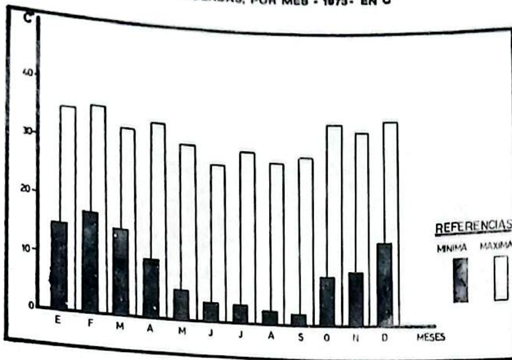
20.p.- TEMPERATURAS MINIMA Y MAXIMA ABSOLUTAS, REGISTRADAS EN POSADAS, POR MES - 1973- EN C°
