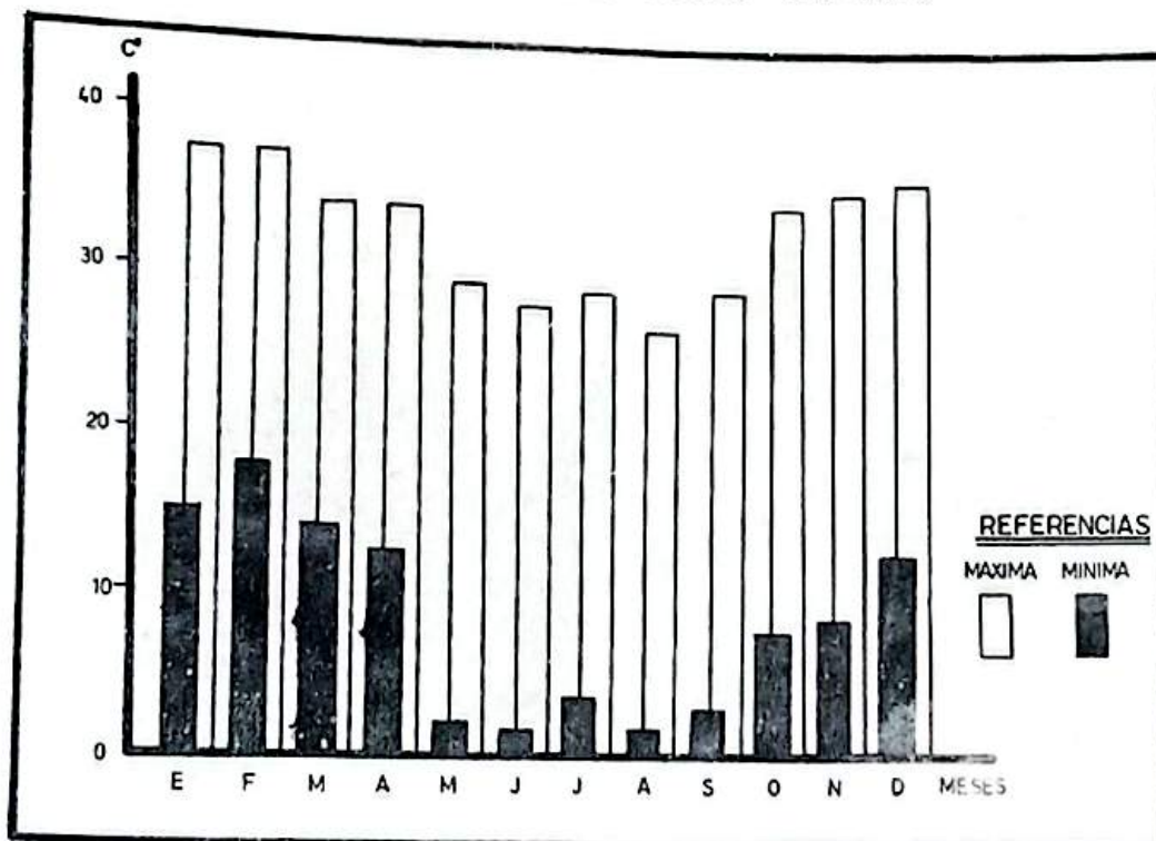
20.q.- TEMPERATURAS MINIMA Y MAXIMA ABSOLUTAS, REGISTRADAS EN MONTECARLO, POR MES - 1973- EN C°
