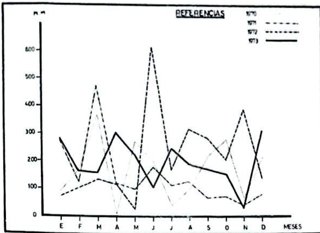
20.o.- EVOLUCION DE LAS PRECIPITACIONES REGISTRADAS EN LA LOCALIDAD DE APOSTOLES, POR MES - 1970-1973 -EN M M
