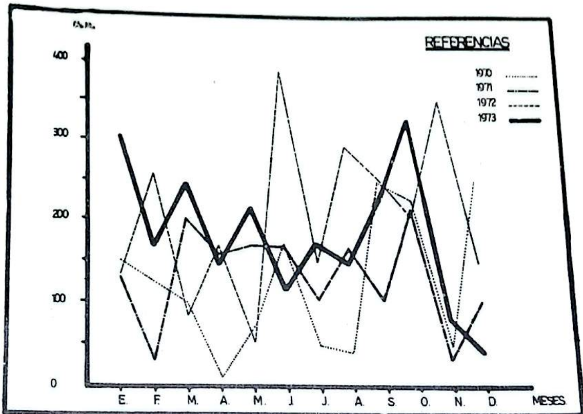
20.B.- EVOLUCION DE LAS PRECIPITACIONES REGISTRADAS EN LA LOCALIDAD DE ELDORADO, POR MES - 1970-1973 - EN M M
