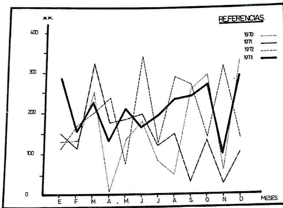
20.d.- EVOLUCION DE LAS PRECIPITACIONES REGISTRADAS EN LA LOCALIDAD DE LINEA BONITA, POR MES - 1970-1973 EN M M
