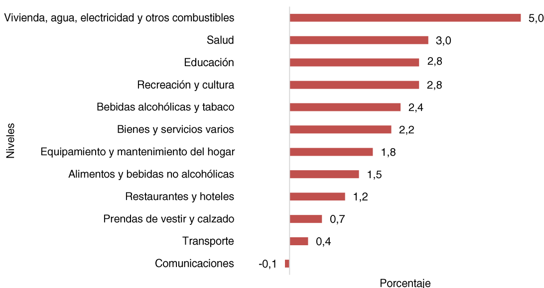
Gráfico 1. IPC variación mensual según divisiones. Región Noreste. Período junio 2026-mayo 2026
