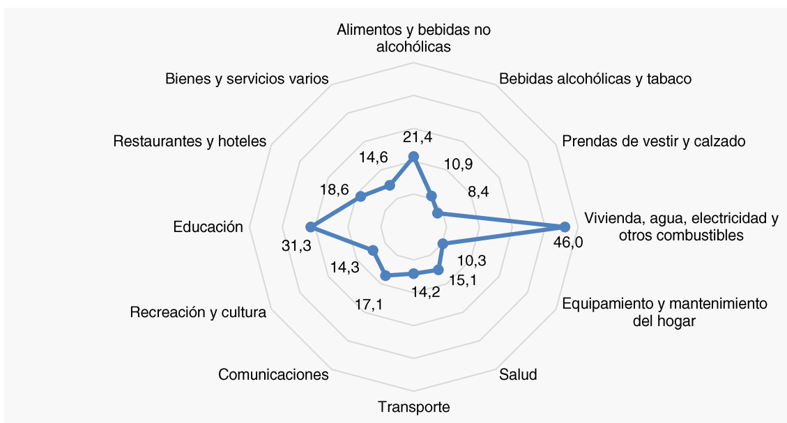
Gráfico 2. IPC variación acumulada anual según divisiones. Región Noreste. Período junio 2026–diciembre 2025
