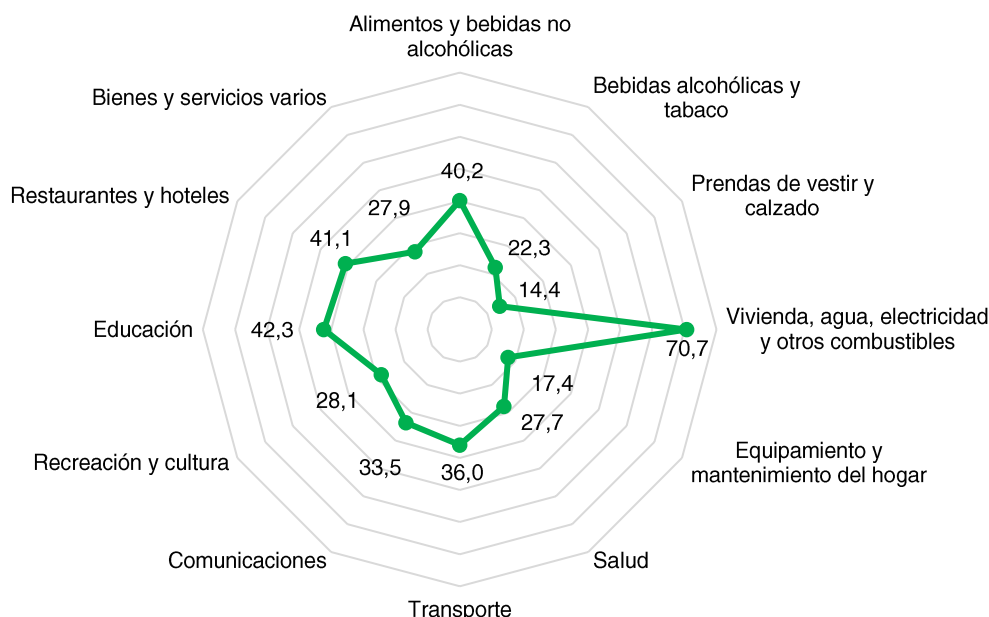
Gráfico 3. IPC variación interanual según divisiones. Región Noreste. Período junio 2026-junio 2025
