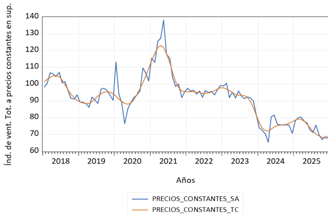
Gráfico 4. Índice de ventas totales a precios constantes. Serie desestacionalizada y tendencia-ciclo. Provincia de Misiones. Año base 2017=100. Enero 2018-diciembre 2025
