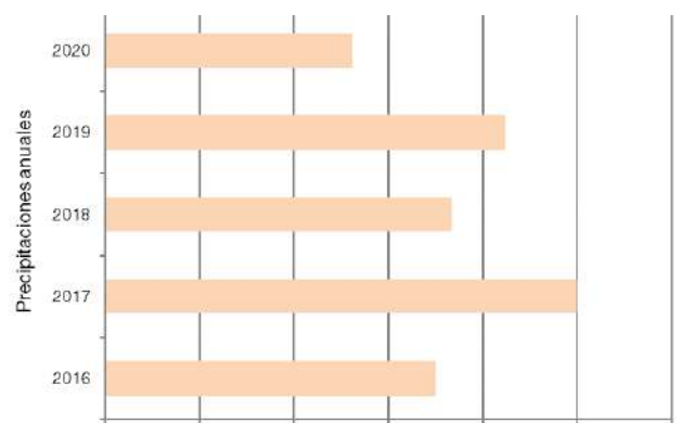
Gráfico 1.2.1 Precipitaciones anuales, en milímetros. Estación meteorológica Posadas. Años 2016-2020
