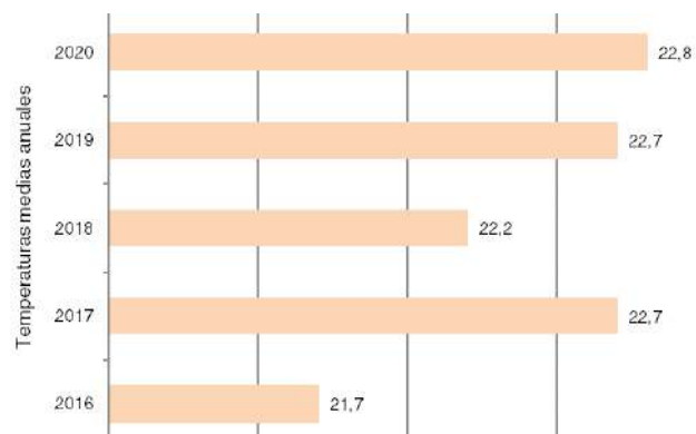
Gráfico 1.2.2 Temperaturas medias anuales por estación meteorológica Posadas. Años 2016-2020
