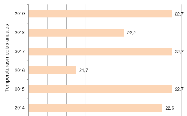
Gráfico 1.2.2 Temperaturas medias anuales. Estación meteorológica Posadas. Años 2014-2019
